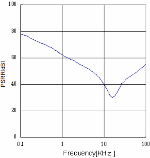
Fig. 32 PSRR ( I_o=0 mA)
