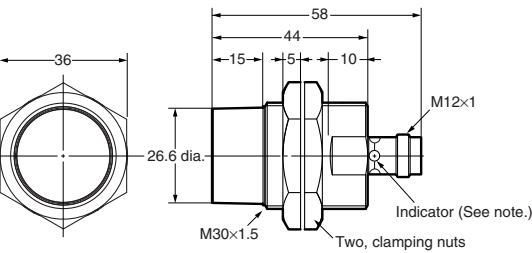
E2A-M30KN20-M1-□□/E2A-S30KN20-M1-□
