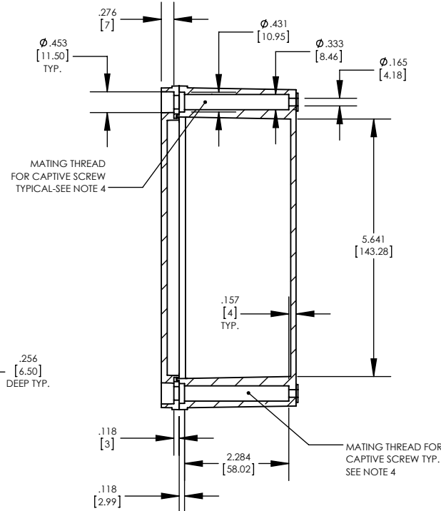
SECTION D-D
