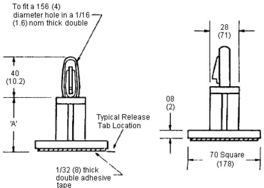
Dimensions : Inches (Millimetres)
