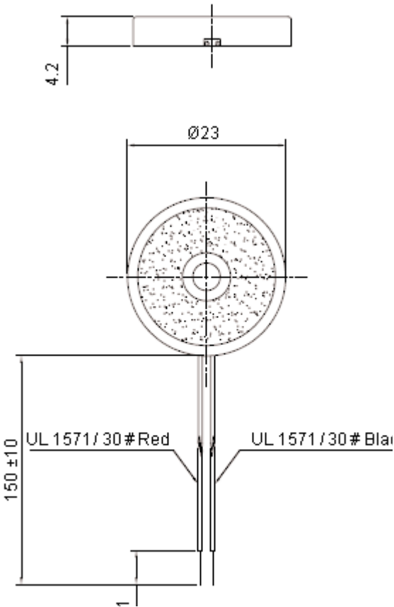
Dimensions : Millimetres
